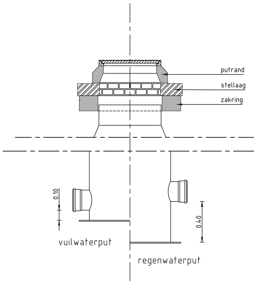
Vuilwater of hemelwater inspectieput schaal 1:20
