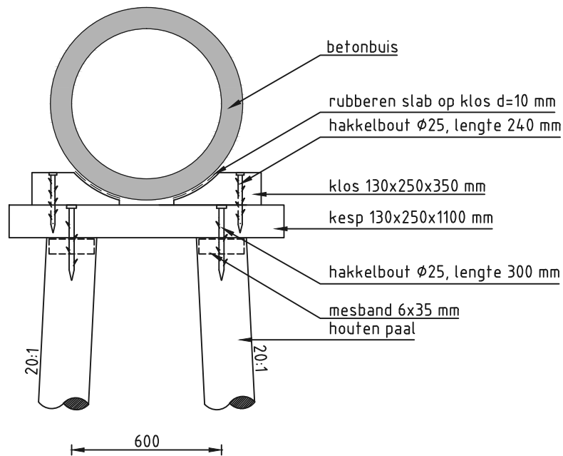
Betonriool \phi 400 en 600 schaal 1:20
