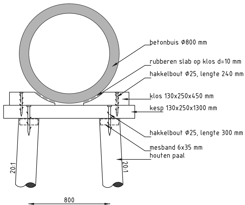
Betonriool \varnothing 800 schaal 1:20
