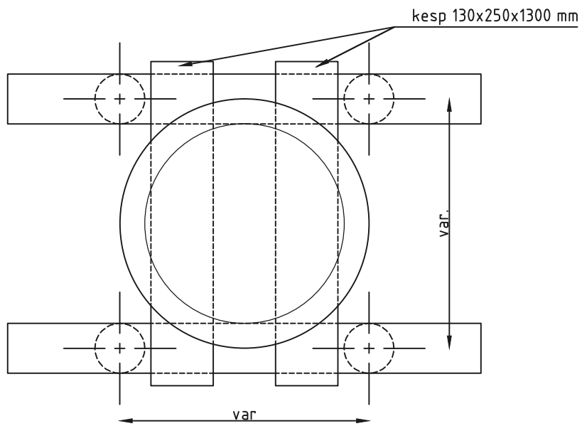
Fundering tpv inspectieput schaal 1:20
